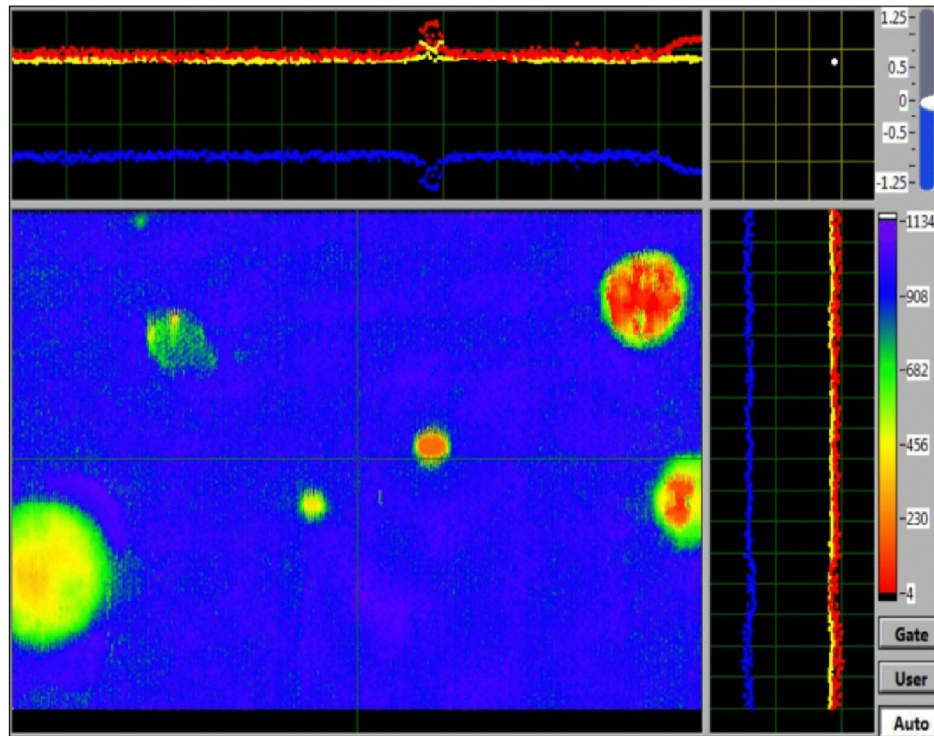
Amplitude display
